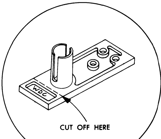
BOTTOM BOLT GUIDE ASSEMBLY FIG. 3B
