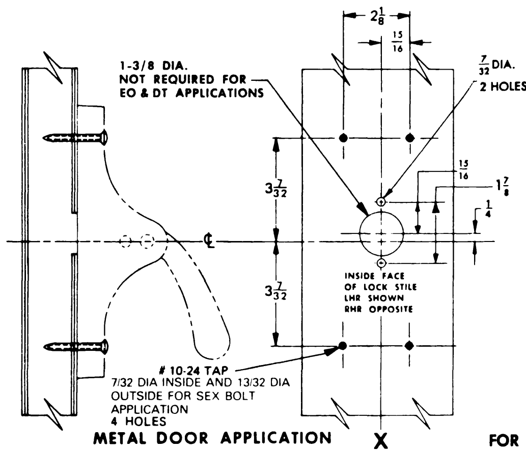
METAL DOOR APPLICATION FIG. 2
